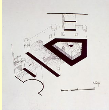
Perspective, vue du dessous, du ravelin (ou barbacane)
